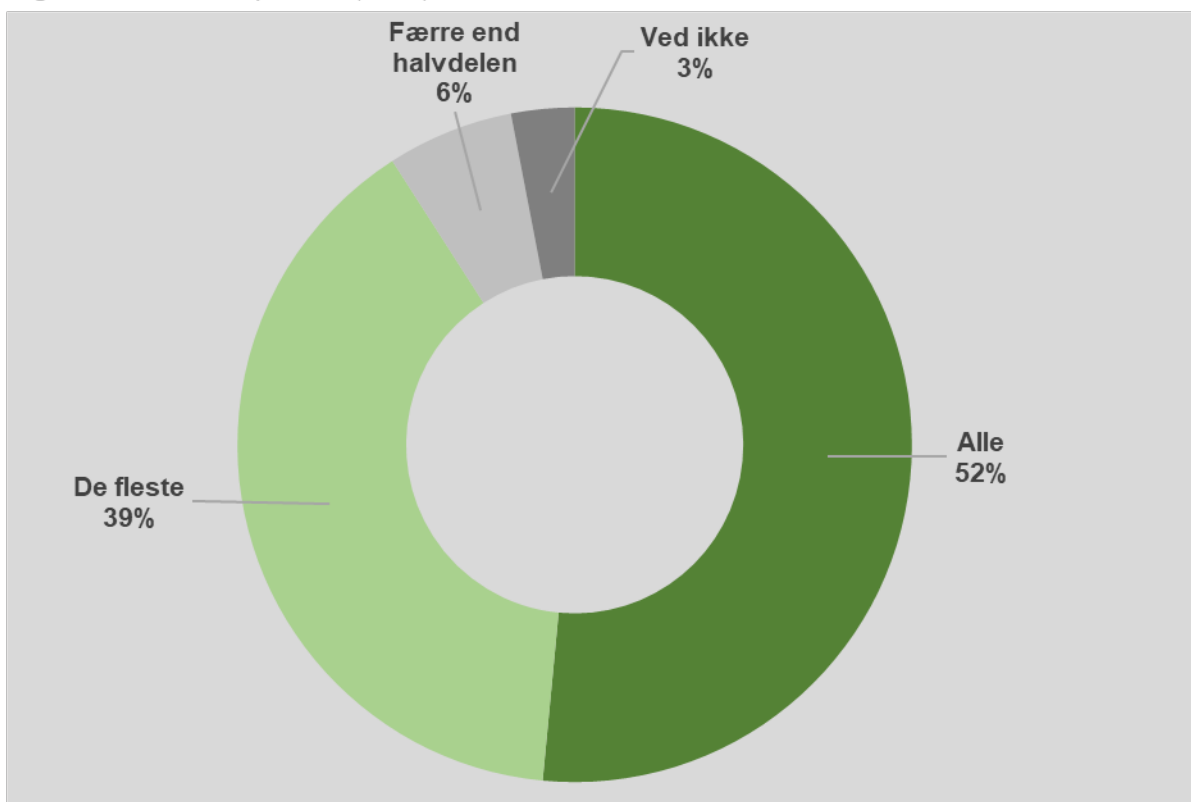
Figur 1. Leveranceopnåelse (n=33)
