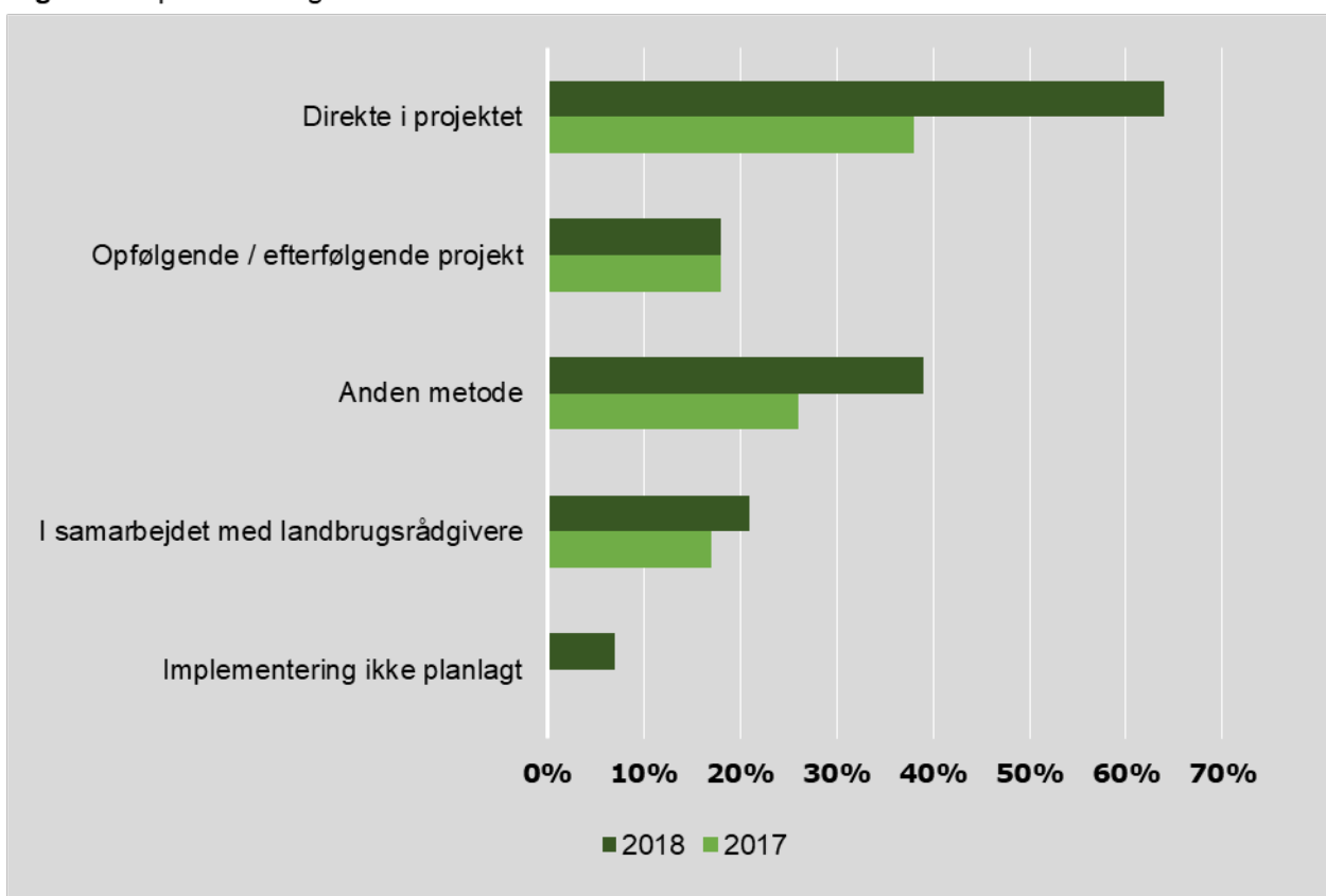
Figur 6. Implementeringsmetode
